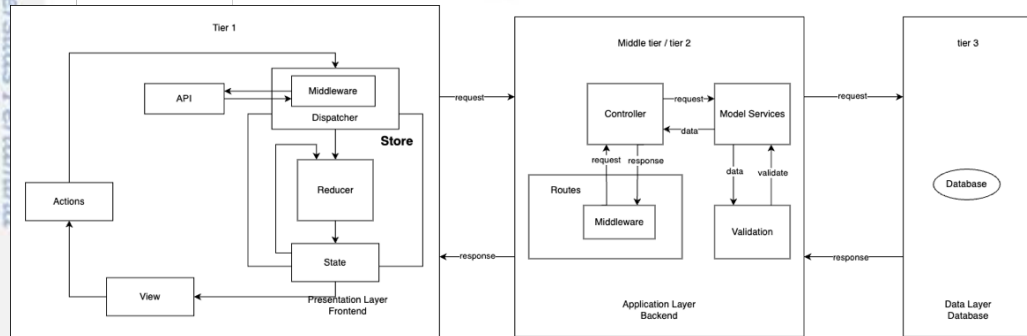
Gambar 10. Penerapan Arsitektur Three-tier layers pada Pengembangan Sistem
