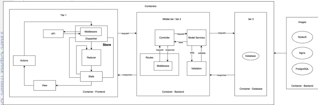
Gambar 11. Skema Arsitektur Perangkat Lunak Menggunakan Docker
