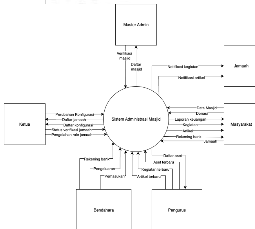
Gambar 13. Context Diagram Sistem Administrasi Masjid
