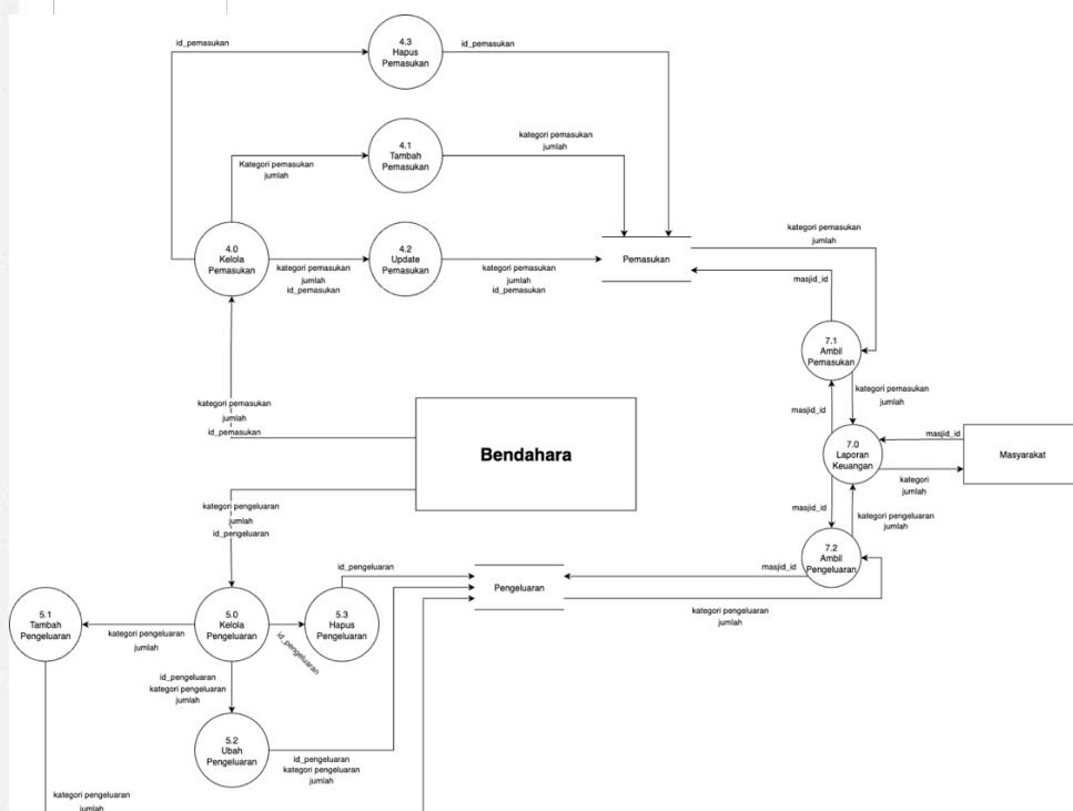
Gambar 16. Data Flow Diagram Level 1 – Kelola Keuangan
