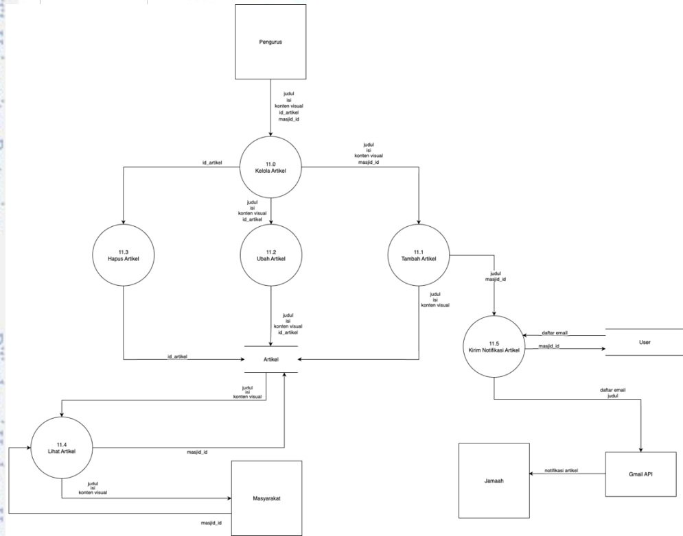
Gambar 20. Data Flow Diagram Level 1 – Kelola Artikel
