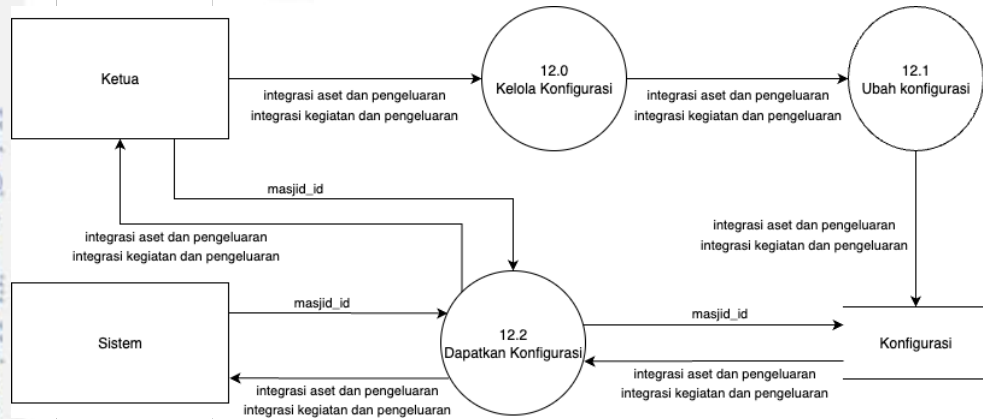
Gambar 21. Data Flow Diagram Level 1 – Kelola Konfigurasi
