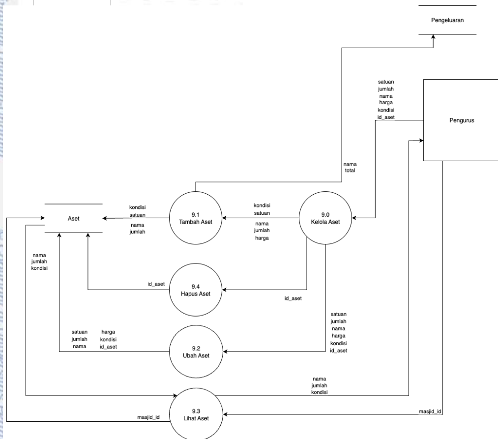
Gambar 18. Data Flow Diagram Level 1 – Kelola Aset
