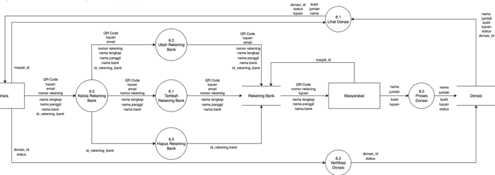
Gambar 17. Data Flow Diagram Level 1 – Kelola Rekening Bank dan Donasi
